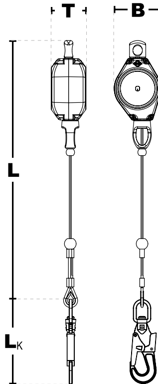
IKV 21 (EN 362:2004-T) mit Fallanzeiger
